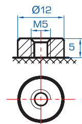
F13 (Schraubanschluss M5)
