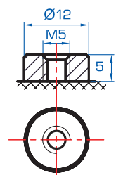
F13 (Schraubanschluss M5)
